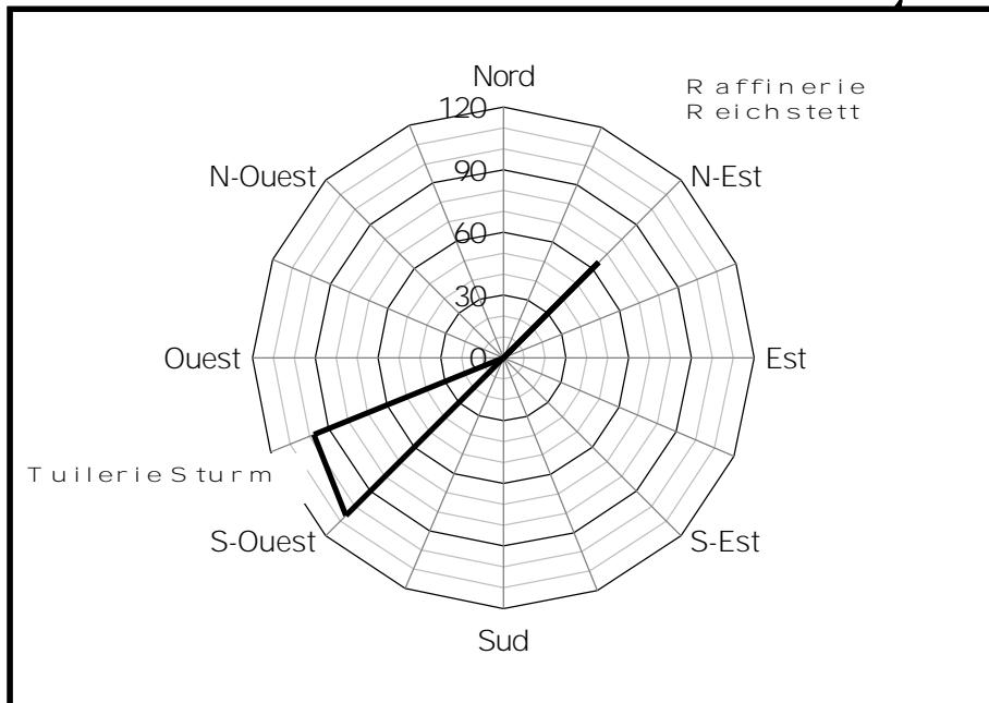
Rose de pollution par le dioxyde de soufre (SO 2 ) déterminée par les mesures effectuées à Oberschaeffolsheim entre le 26 février et le 15 mars 2000. L'échelle utilisée indique la concentration de SO 2 en µg/m 3 .
